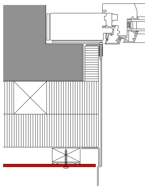
Fensterleibung (Metallabdeckung)
