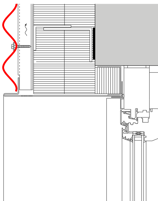
Fenstersturz
