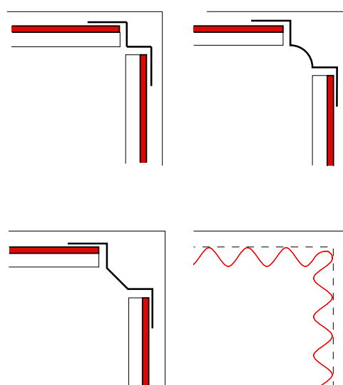
Ausführung von Innenecken
