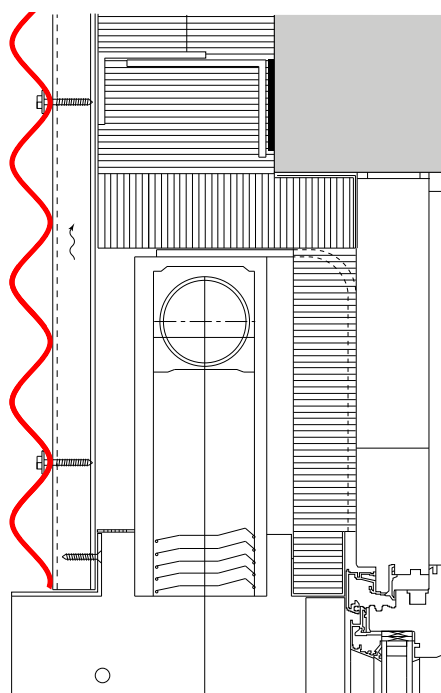
Fenstersturz mit Sonnenschutz
