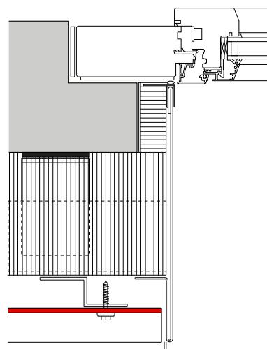
Fensterleibung (Metallabdeckung)
