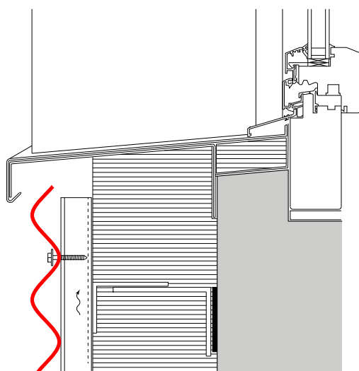
Fensterbrüstung
